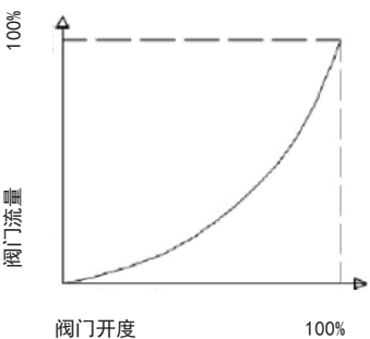
等百分比流量特性
