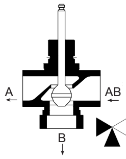
DN15-DN50三通分流接法
