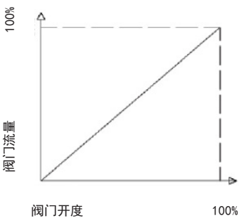
等线性流量特性
