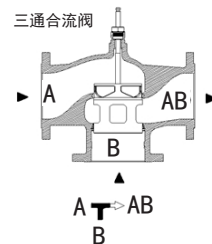
三通合流接法
