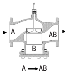
DN32~DN200二 通阀体
