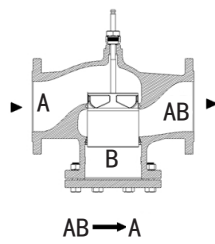
DN15~DN25 二通阀体
