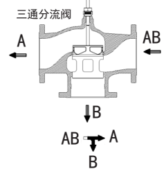
三通分流接法
